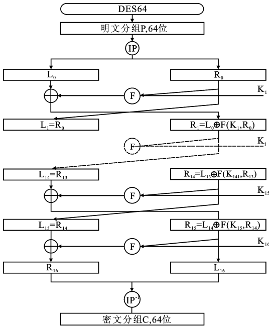
图 1 DES 加密流程
