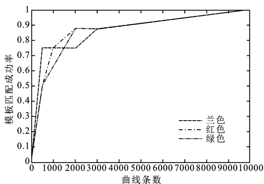
图 3 模板匹配成功率曲线
